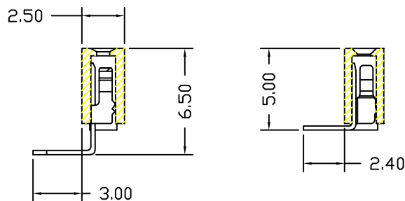
SCALE 1:1 SECTION A-A
